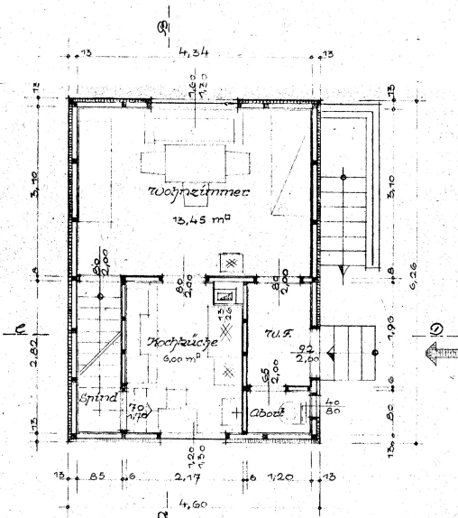
Erdgeschoss
