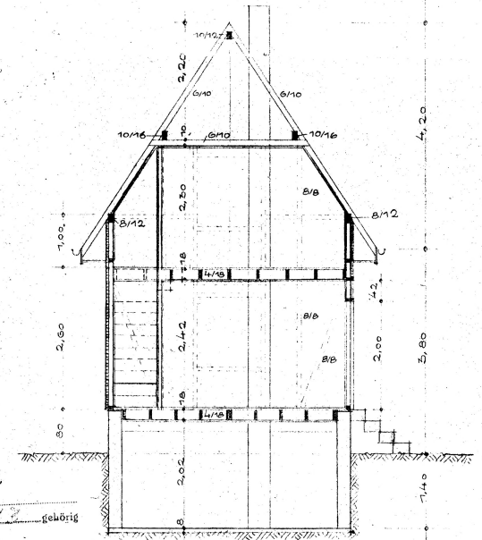
Schnitt e-D
