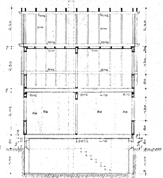
Schnitt A-B
